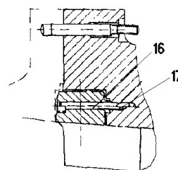
DETAIL Y PART. Y
