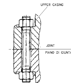
SECTION D-D SEZIONE D-D
