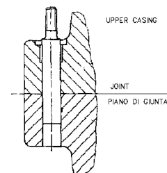
SECTION D-D SEZIONE D-D
